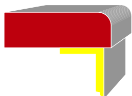
Leštěný výřez pro spodní dřež s hranou R8 nebo A30
